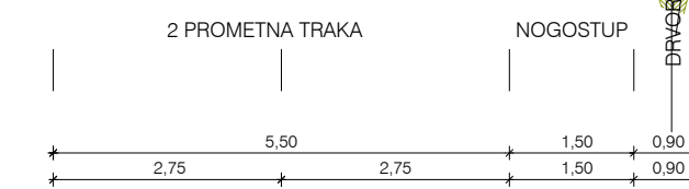
PRESJEK D-D, MJ 1:100
