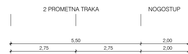
PRESJEK C-C
