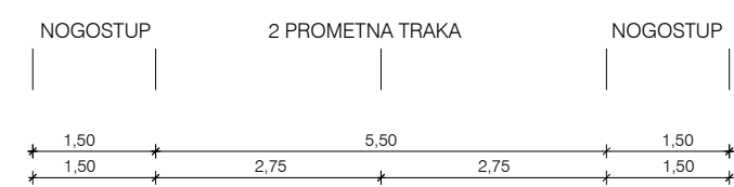
PRESJEK A-A
